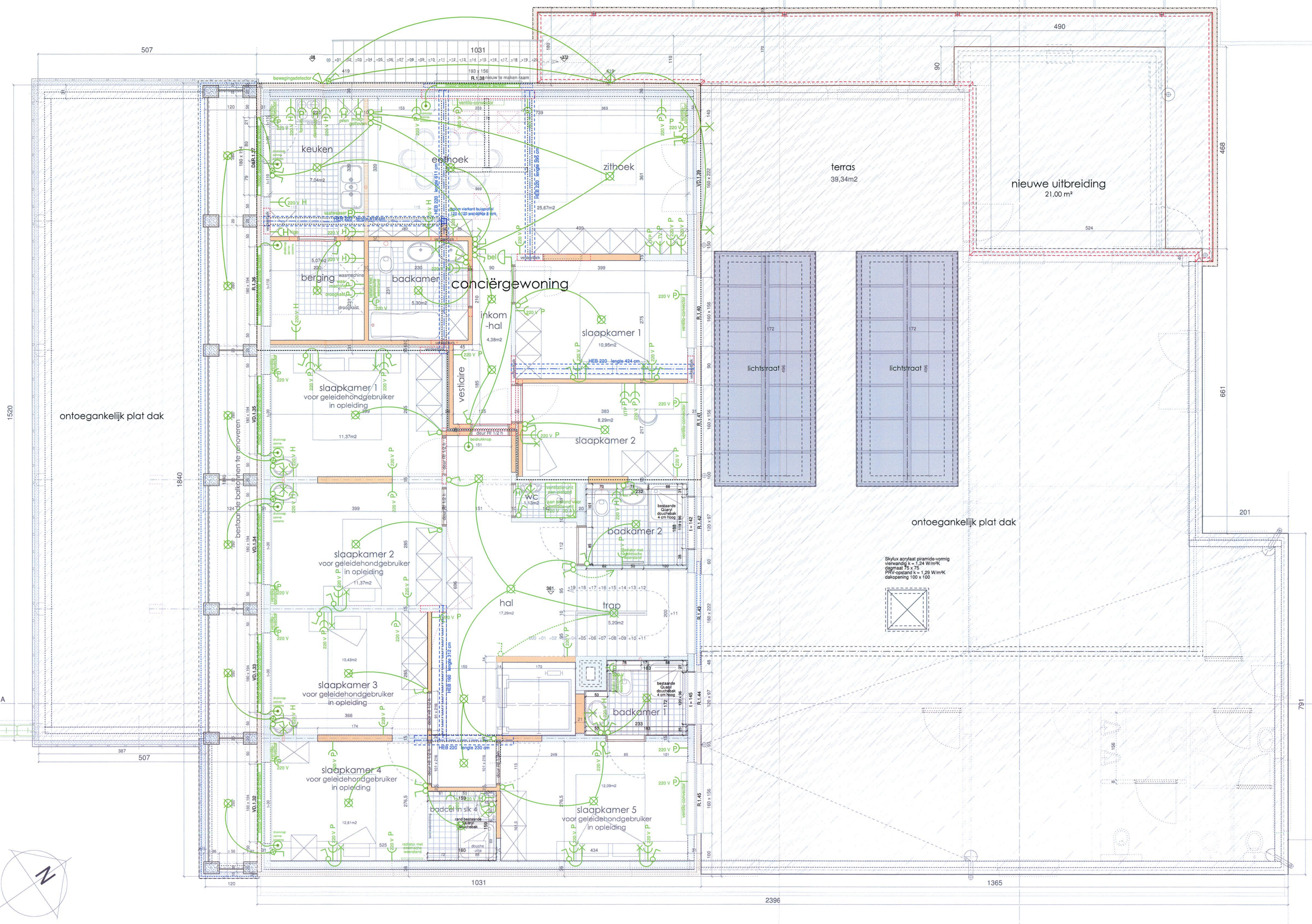
EERSTE VERDIEPING schaal 1/50
